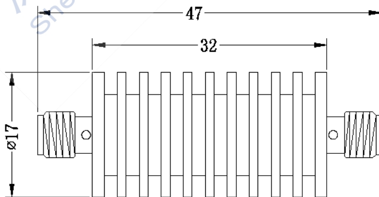
尺寸单位: mm 外形尺寸公差: \pm 2\%
